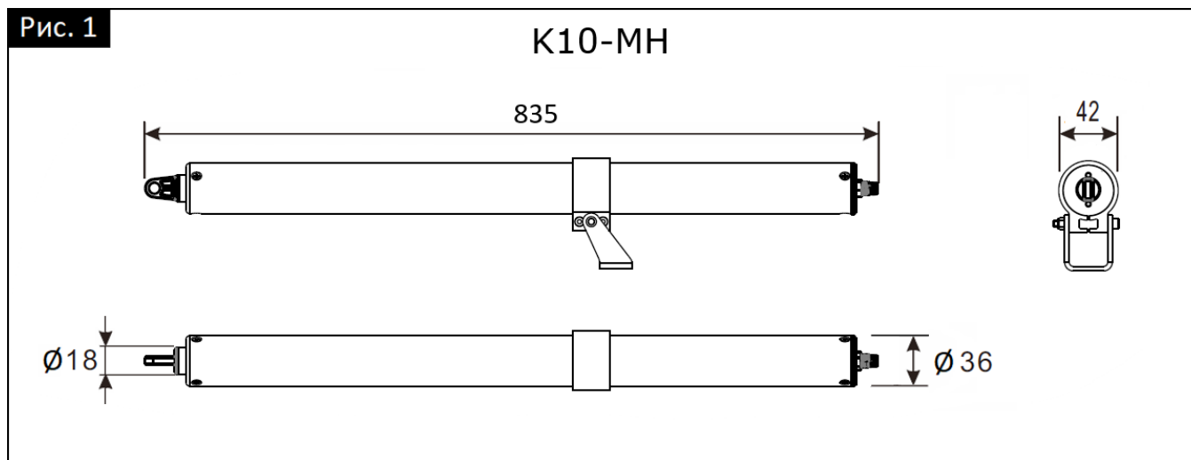
Рис. 1. Габаритные размеры привода K10-MH 24В 400 мм.
